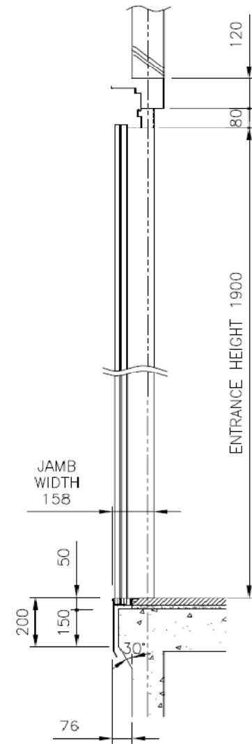
A-A SECTION
